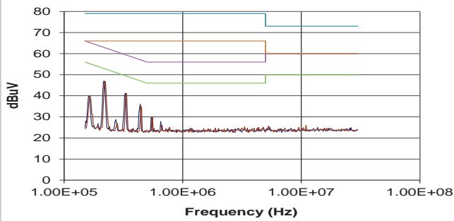
MEV3S0512SC
