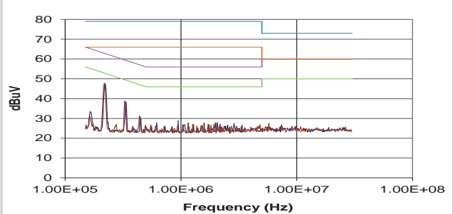
MEV3S1209SC
